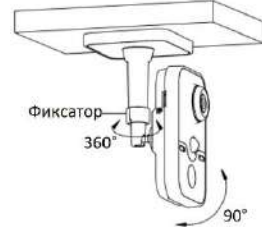
Рисунок 1-27 Настройка угла наблюдения камеры
