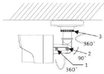
Рисунок 1-2 Настройка угла наблюдения камеры
