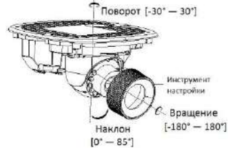
Рисунок 1-25 Настройка угла наблюдения камеры
